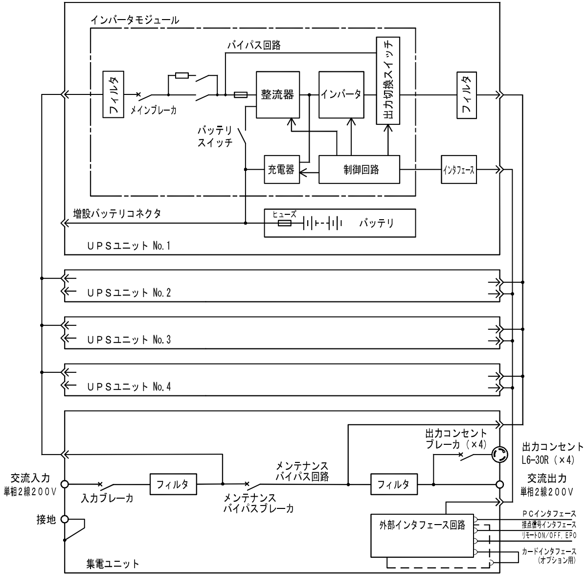
上図は UPSS-200X3-010RM の回路系統図です。
