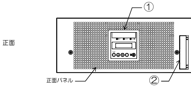
UPSユニット
