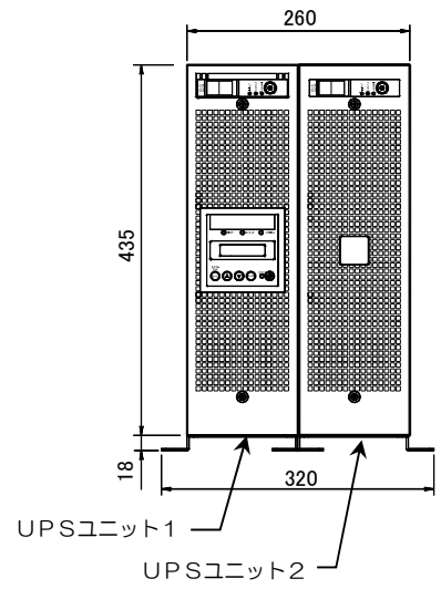
床固定寸法図
