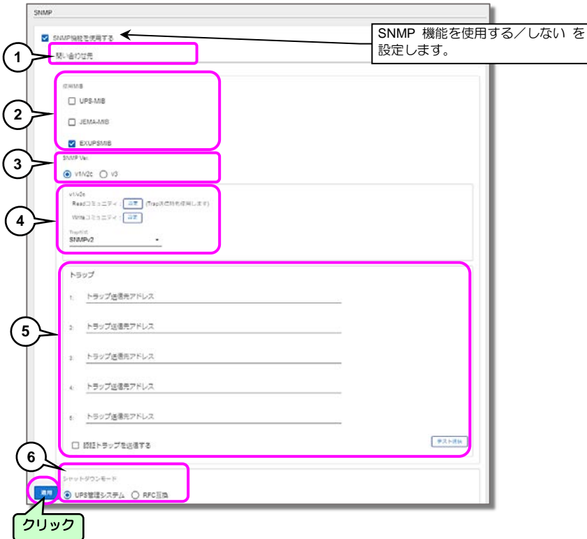
「SNMP」画面
