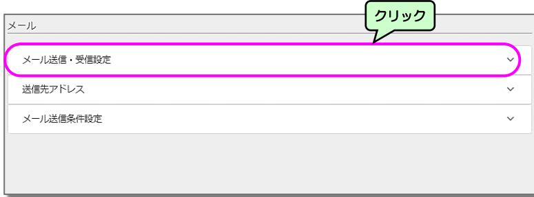
「メール」画面
