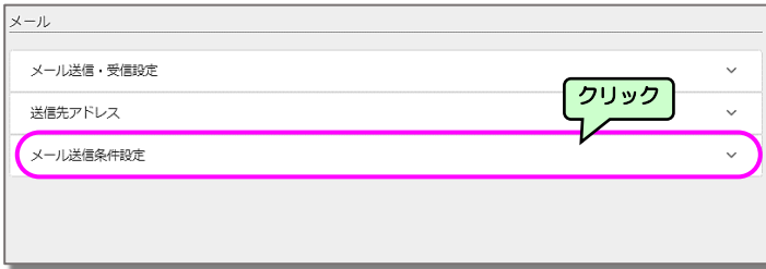
「メール」画面
