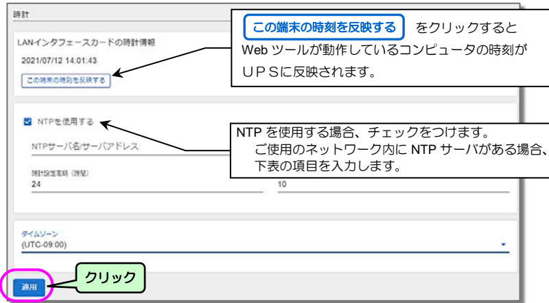
「時計」画面
